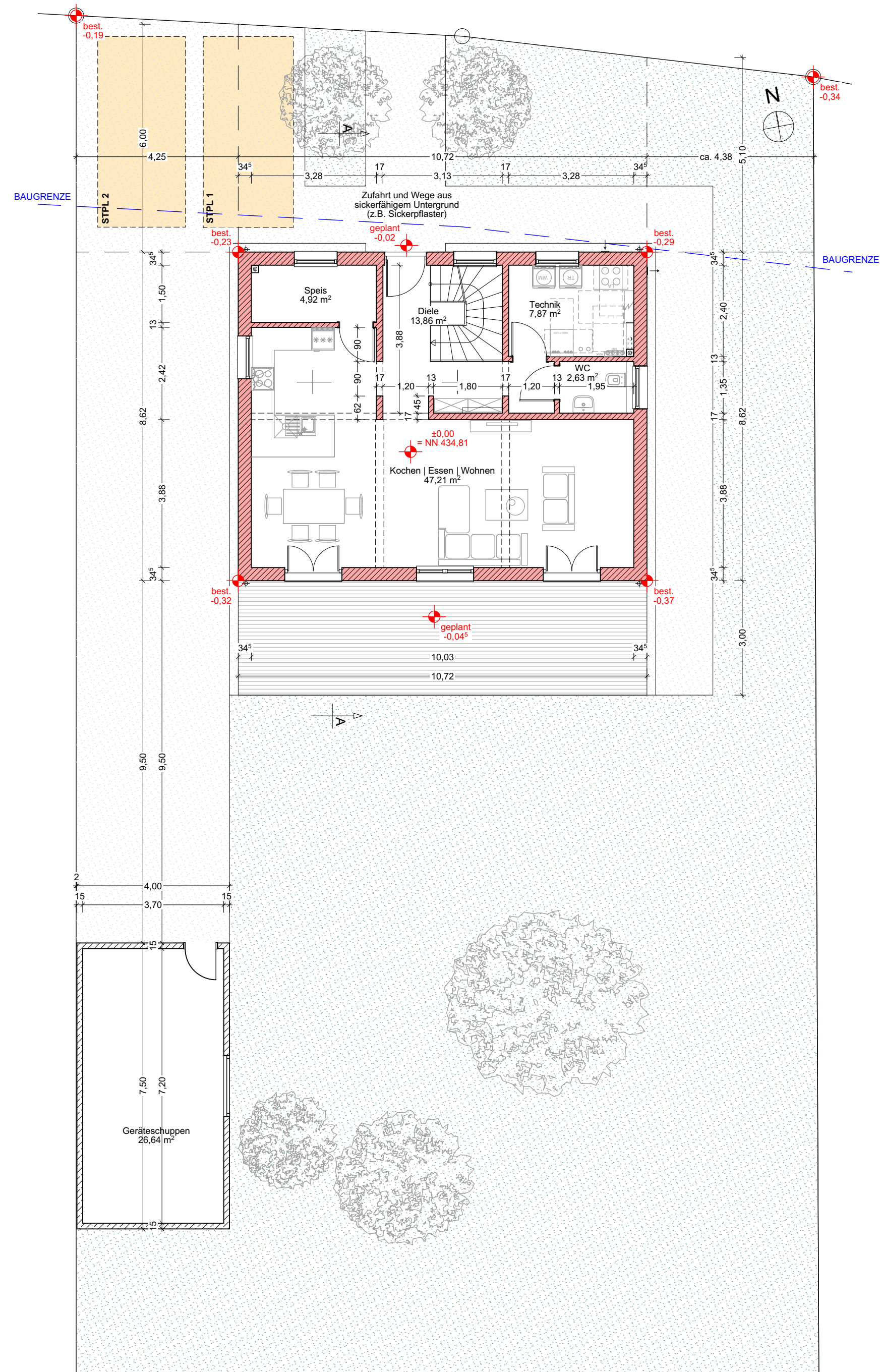
GRUNDRISS EG
