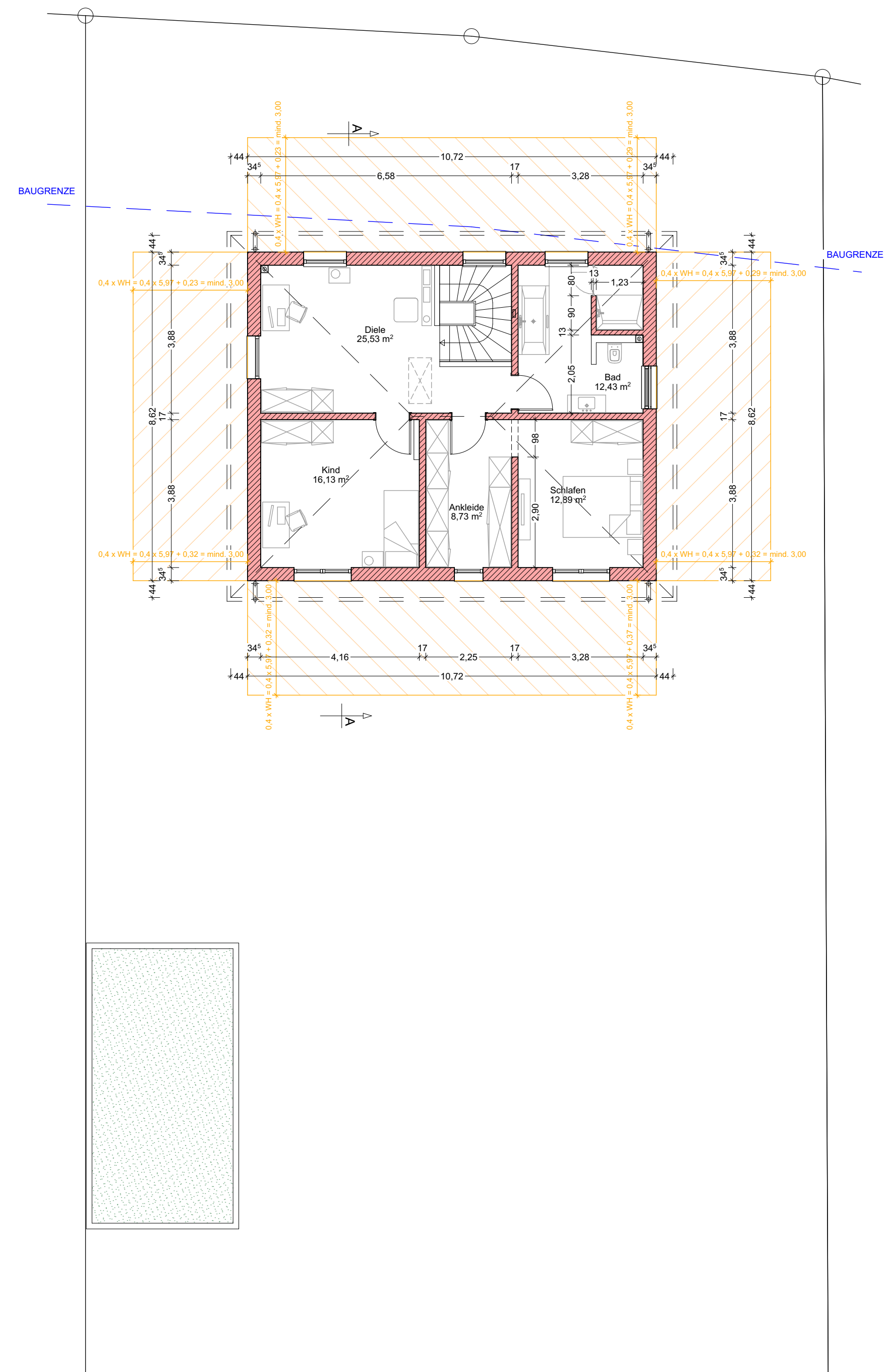
GRUNDRISS OG
