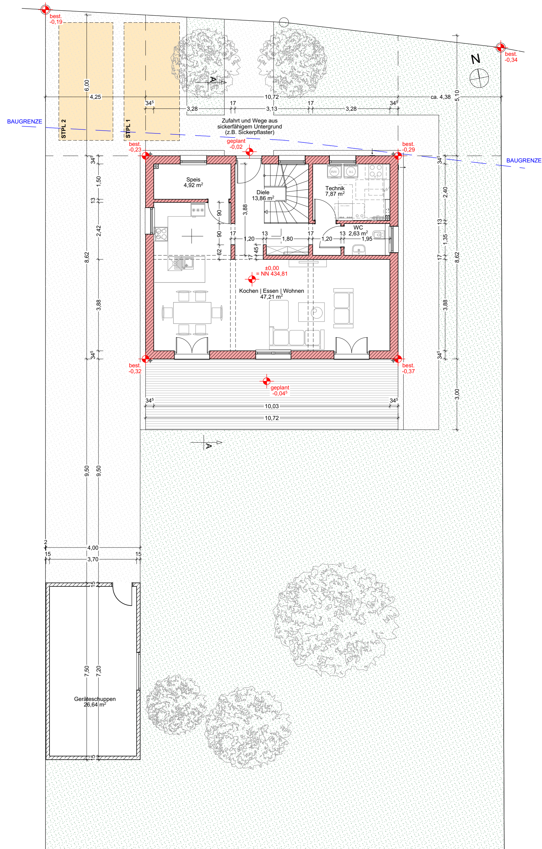
GRUNDRISS EG
