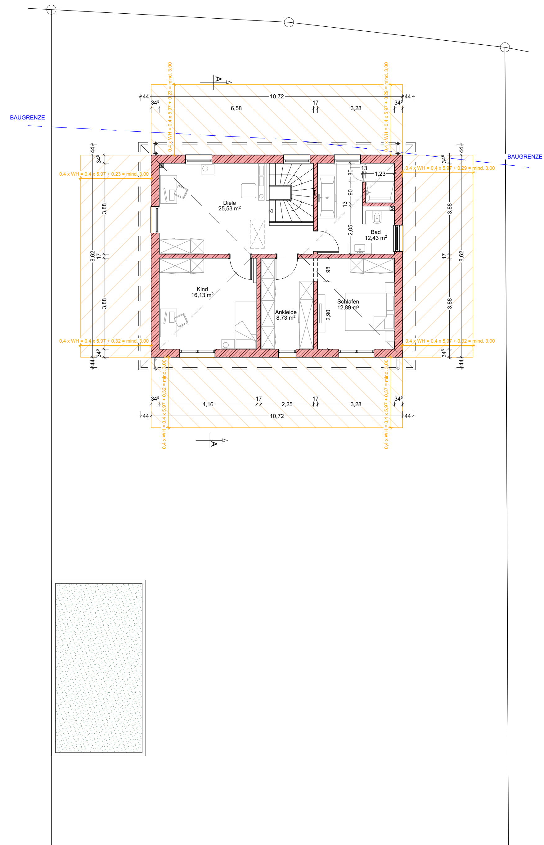
GRUNDRISS OG
