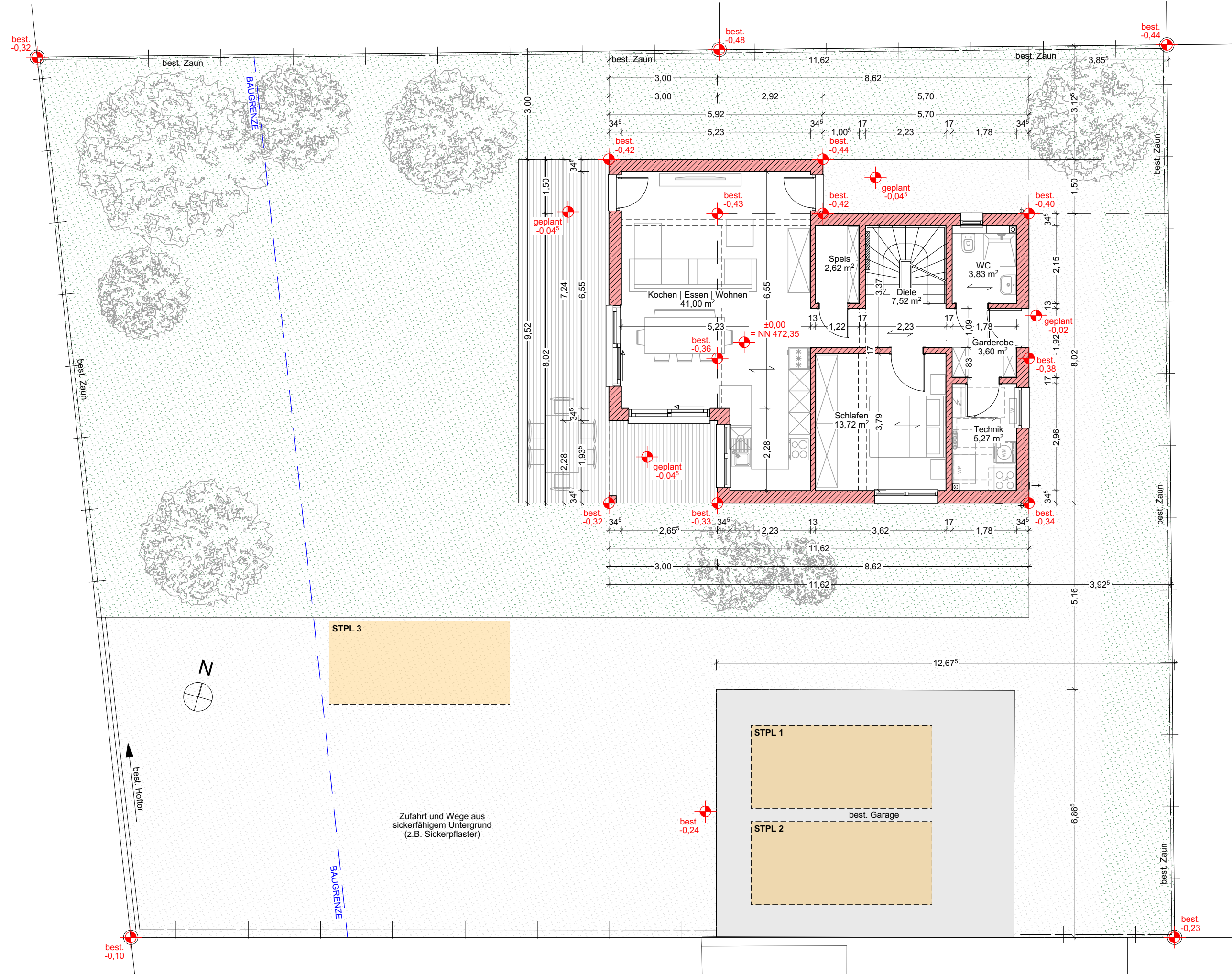
GRUNDRISS EG
