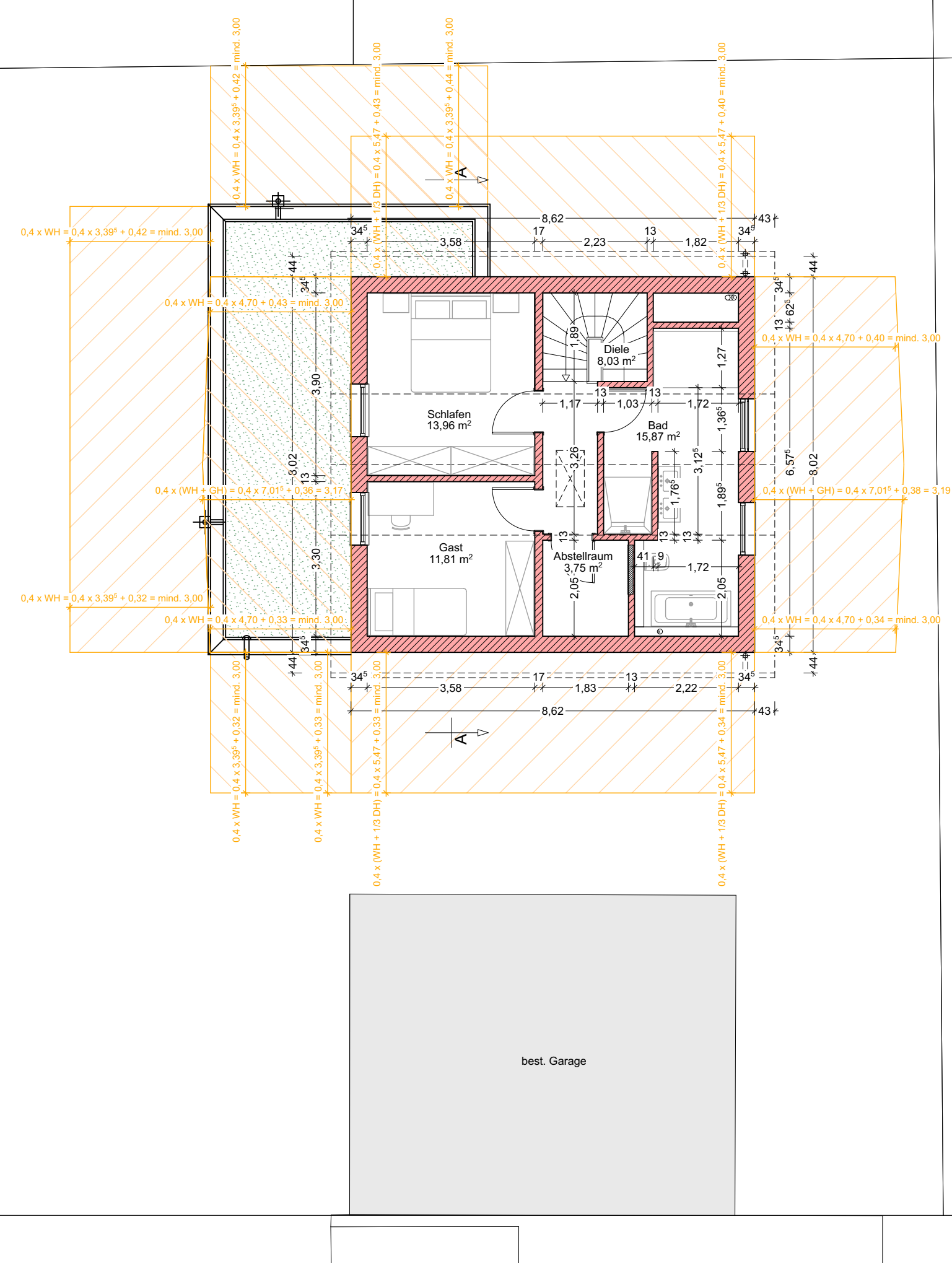
GRUNDRISS OG
