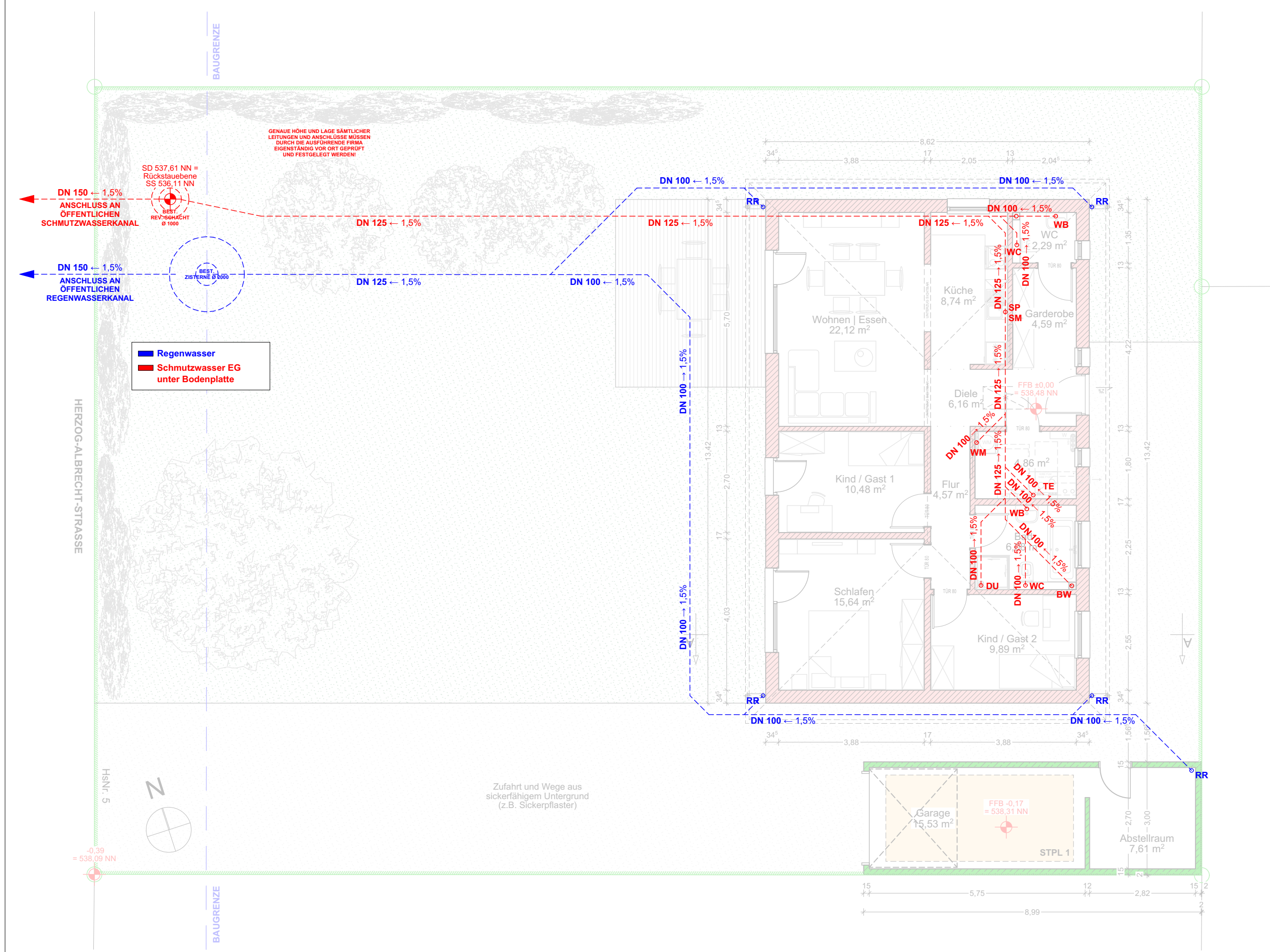
GRUNDRISS EG - ENTWÄSSERUNG
