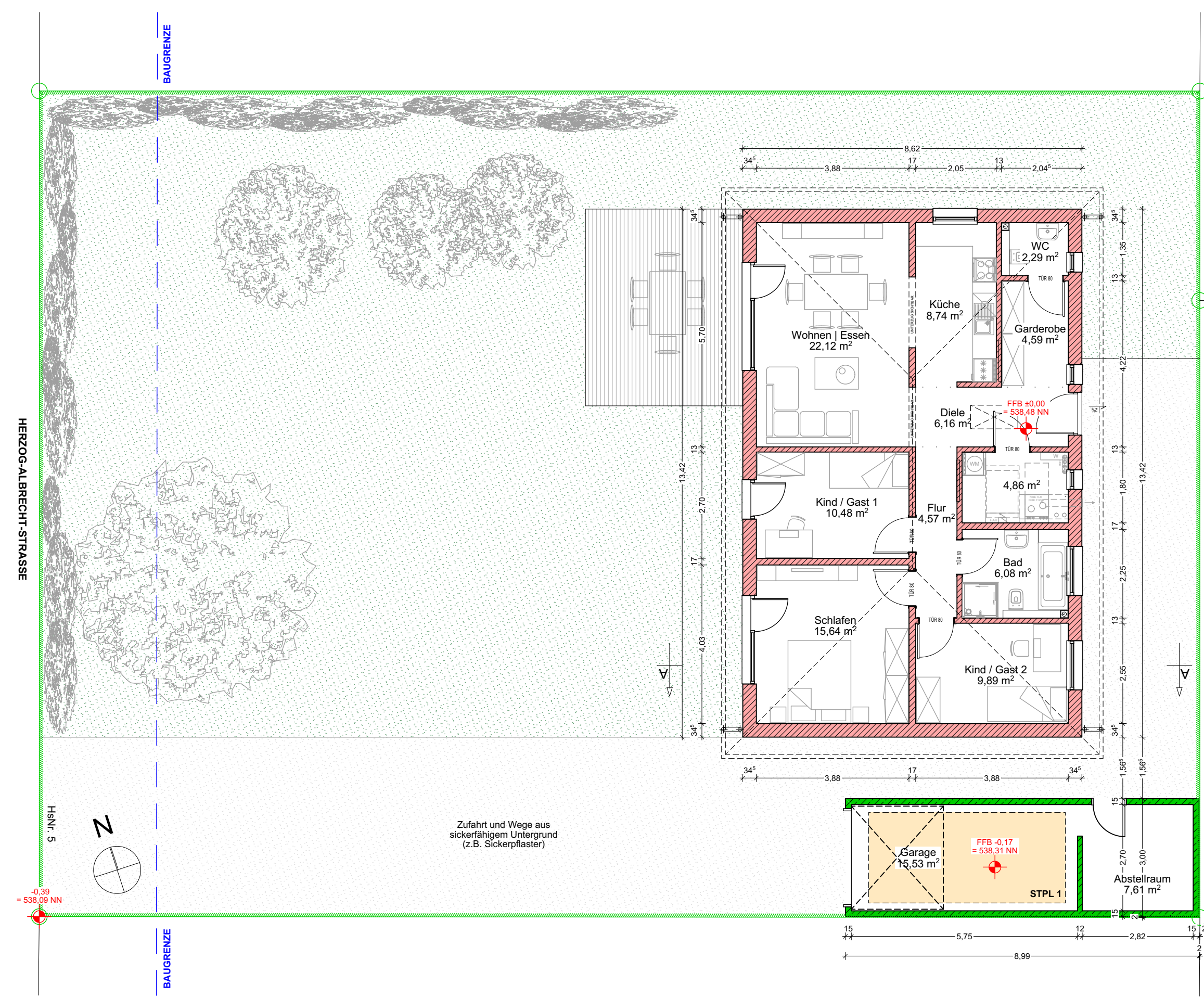
GRUNDRISS EG
