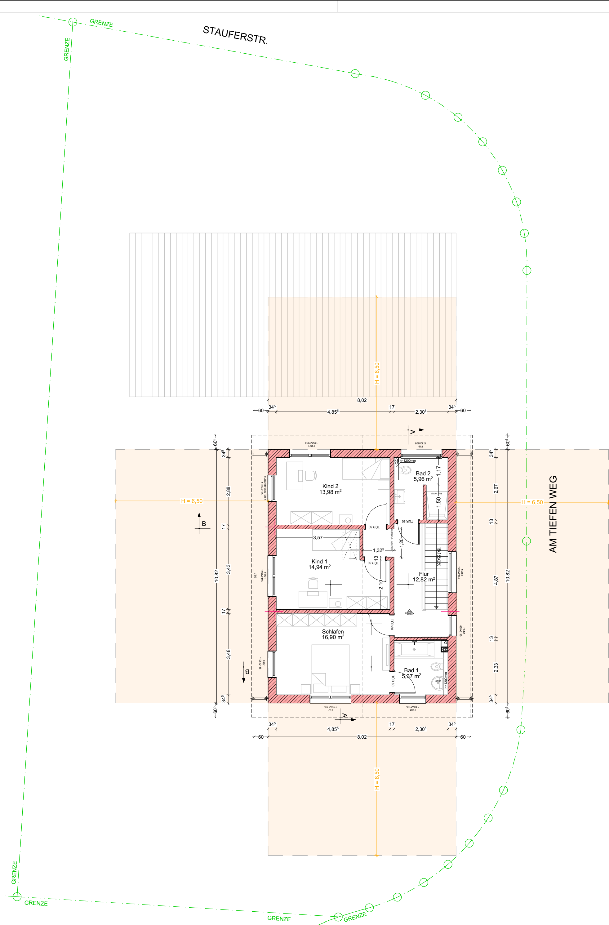
GRUNDRISS OG - ABSTANDSFLÄCHEN
