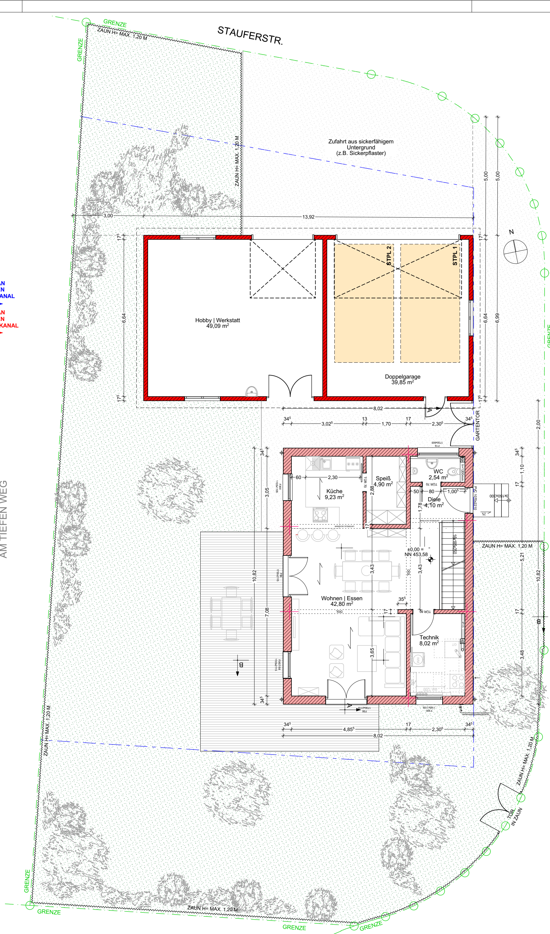
GRUNDRISS EG
