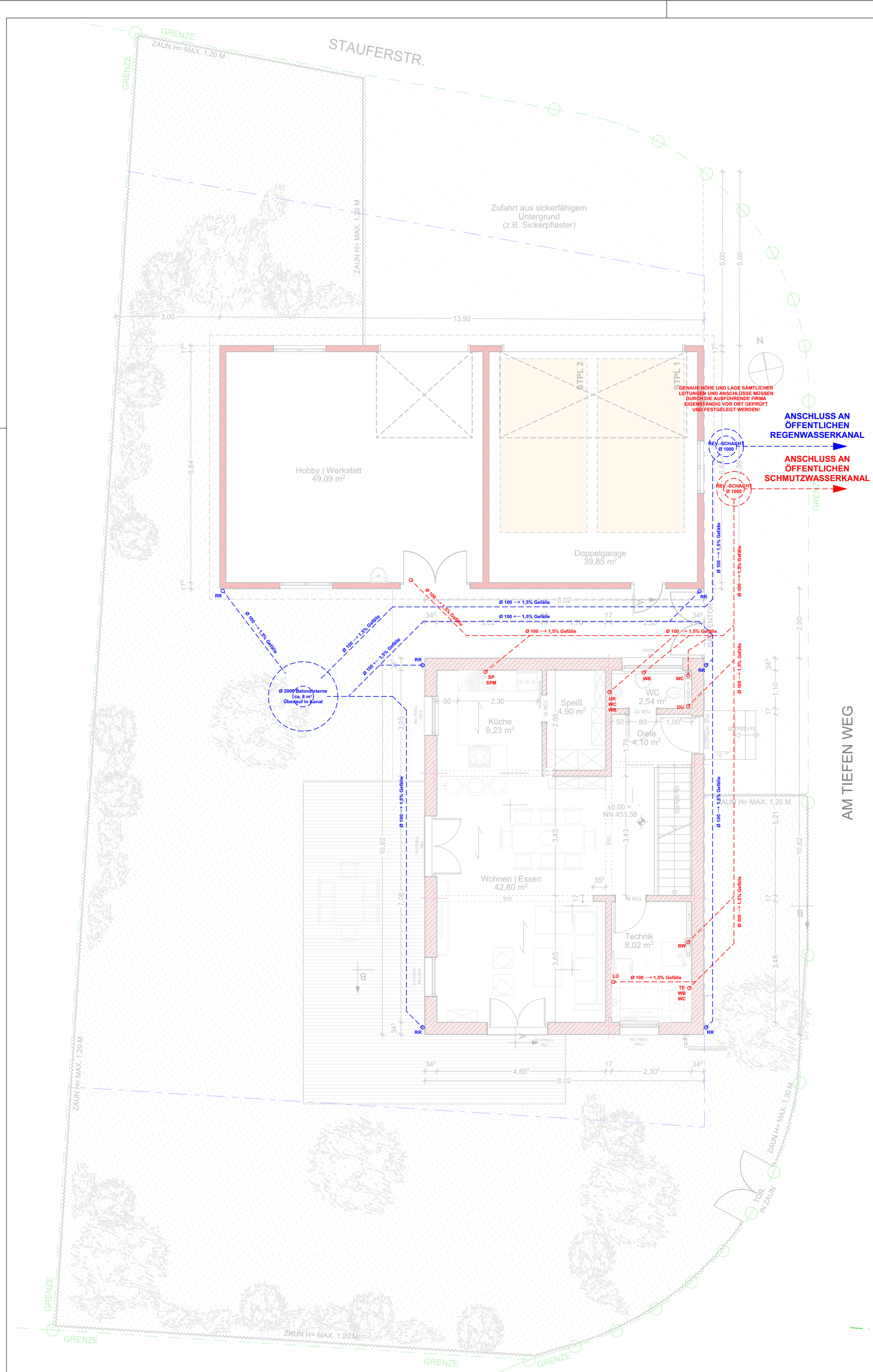
GRUNDRISS EG - ENTWÄSSERUNG
